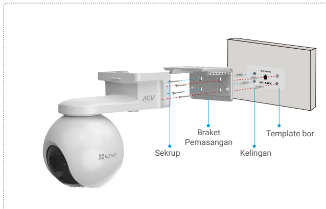
Gbr. 2 Pemasangan pada Dinding
