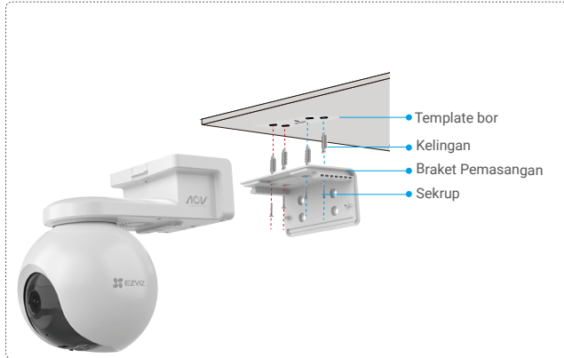
Gbr. 1 Pemasangan pada Plafon
